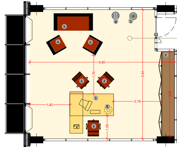
Tipologia DIREZIONALE - UFFICIO DIRIGENTE - Mq 37,04
