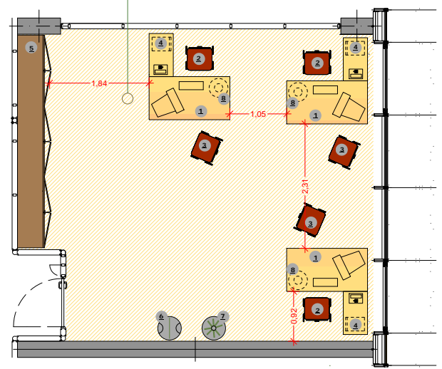
Tipologia 3 scrivanie - UFFICIO OPERATIVO - (tipo B) Mq 36,63
