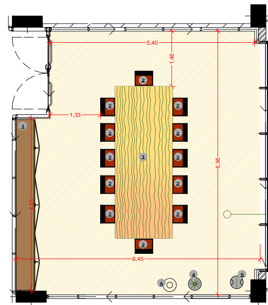
Tipologia SALA RIUNIONI - (tipo A) Mq 42.43
