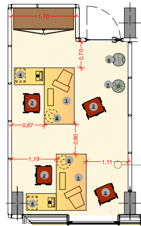
Tipologia 2 scrivanie - UFFICIO OPERATIVO - (tipo C) Mq 15,51
