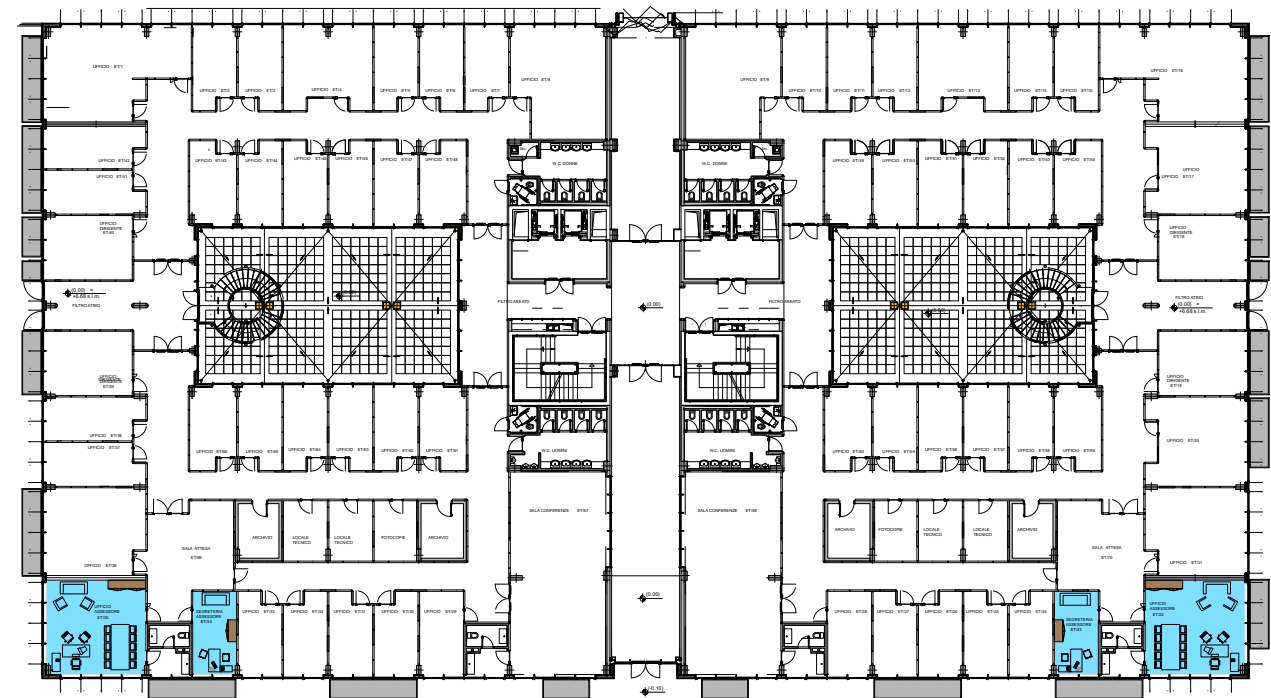
CORPO E - PIANO TERRA SCALA 1:500
