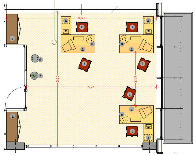
Tipologia 3 scrivanie - UFFICIO OPERATIVO - (tipo A) Mq 35,54
