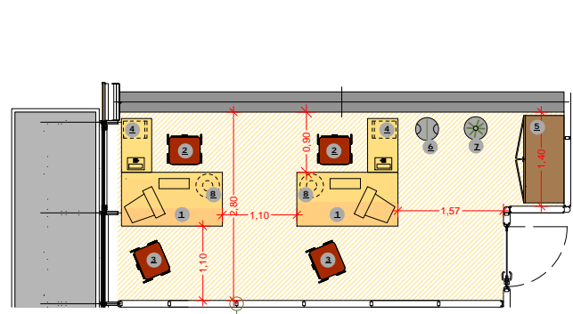
Tipologia 2 scrivanie - UFFICIO OPERATIVO - (tipo A) Mq 17,22
