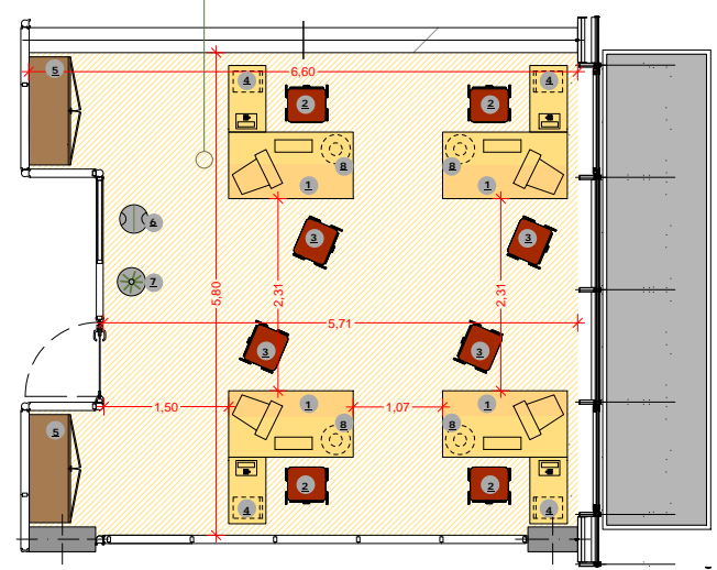
Tipologia 4 scrivanie - UFFICIO OPERATIVO - (tipo B) Mq 35,54
