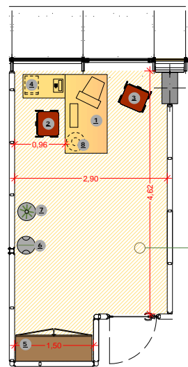
Tipologia 1 scrivania - UFFICIO OPERATIVO - (tipo B) Mq 14,63
