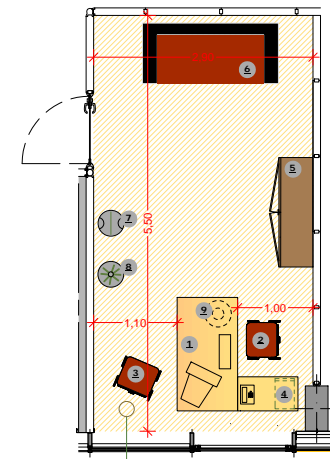
Tipologia 1 scrivania - UFFICIO SEGRETERIA/ COORDINATORE - Mq 15.89
