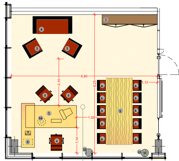
Tipologia 1 scrivania - UFFICIO COORDINATORE/ ASSESSORE - Mq 41.00
