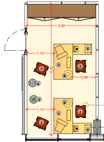
Tipologia 2 scrivanie - UFFICIO OPERATIVO - (tipo D) Mq 15,84
