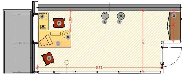
Tipologia 1 scrivania - UFFICIO OPERATIVO - (tipo A) Mq 17,22
