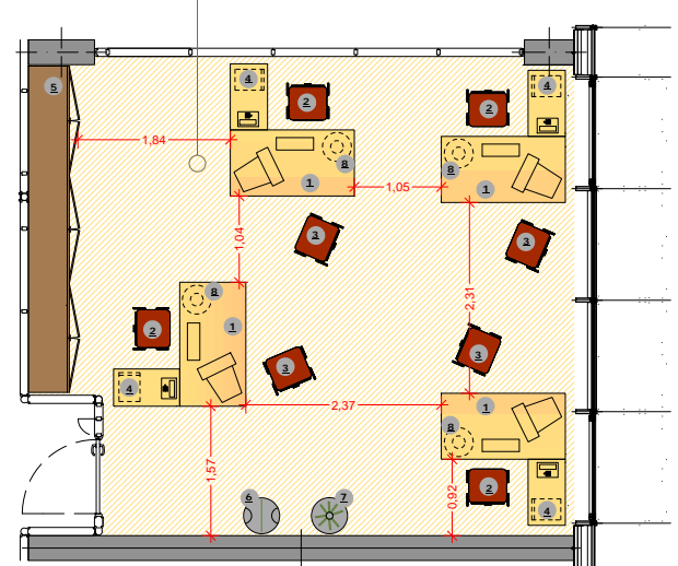
Tipologia 4 scrivanie - UFFICIO OPERATIVO - (tipo B) Mq 36,63
