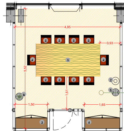
Tipologia SALA RIUNIONI - (tipo B) Mq 24.91
