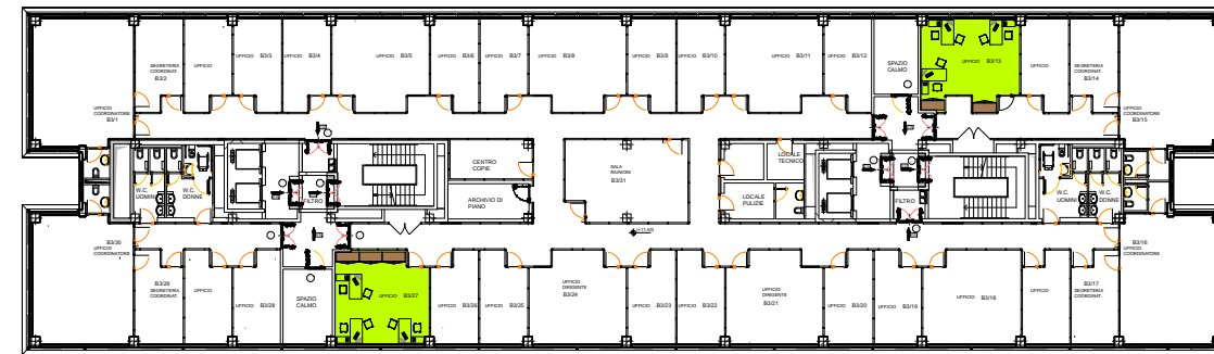
CORPO B - PIANO 3°
