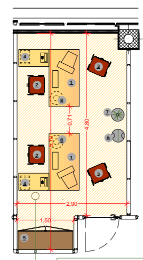
Tipologia 2 scrivanie - UFFICIO OPERATIVO - (tipo A) Mq 15,16
