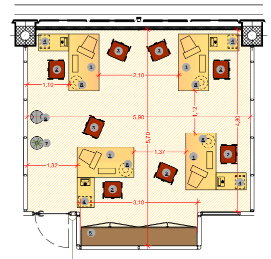
Tipologia 4 scrivanie - UFFICIO OPERATIVO - (tipo A) Mq 30,95
