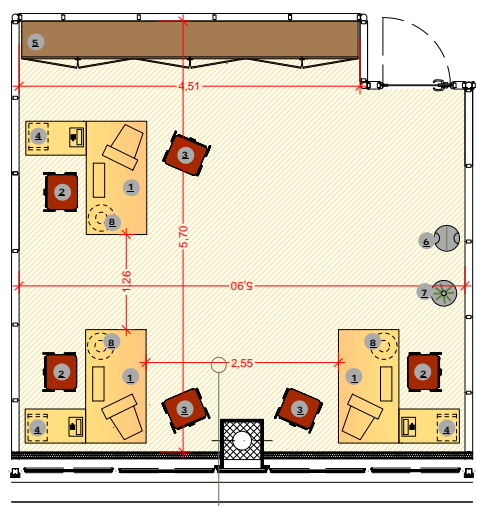
Tipologia 3 scrivanie - UFFICIO OPERATIVO - (tipo B) Mq 32,16
