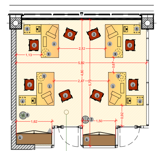
Tipologia 4 scrivanie - UFFICIO OPERATIVO - (tipo B) Mq 30,96
