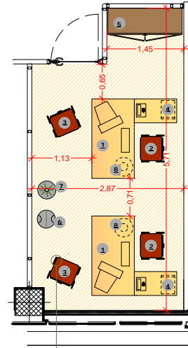
Tipologia 2 scrivanie - UFFICIO OPERATIVO (tipo B)- Mq 14,76
