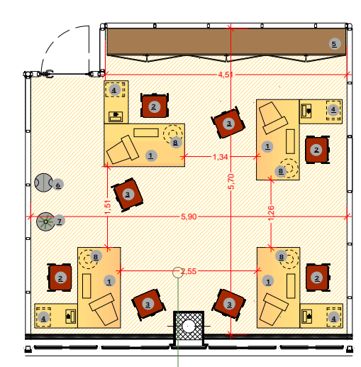
Tipologia 4 scrivanie - UFFICIO OPERATIVO - (tipo C) Mq 32,16
