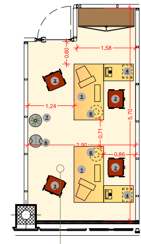
Tipologia 2 scrivanie - UFFICIO OPERATIVO - (tipo C) Mq 15.25
