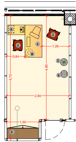
Tipologia 2 scrivanie - UFFICIO OPERATIVO - (tipo A) Mq 15,16
