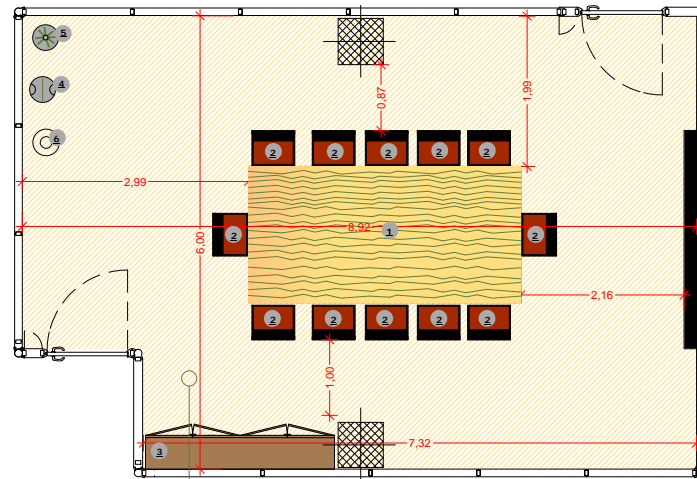
Tipologia SALA RIUNIONI - Mq 50,33
