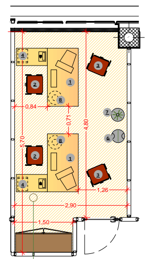
Tipologia 2 scrivanie - UFFICIO OPERATIVO - (tipo A) Mq 15.16
