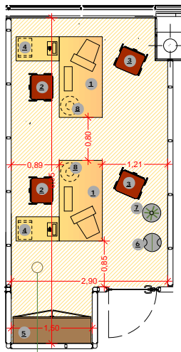
Tipologia 2 scrivanie - UFFICIO OPERATIVO - (tipo A) Mq 15,93
