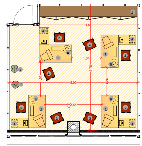
Tipologia 4 scrivanie - UFFICIO OPERATIVO - (tipo B) Mq 32,16
