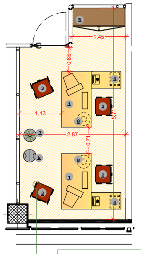
Tipologia 2 scrivanie - UFFICIO OPERATIVO (tipo B) - Mq 14,76
