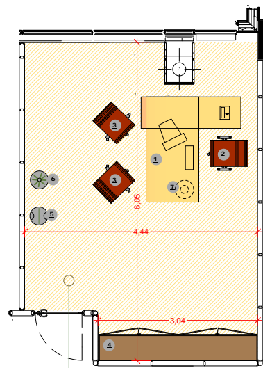
Tipologia DIREZIONALE - UFFICIO DIRIGENTE - Mq 25,11
