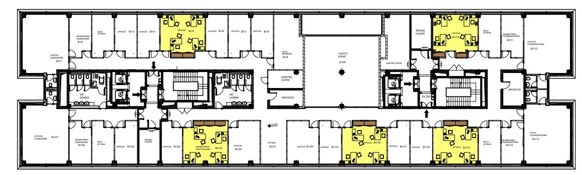
CORPO B - PIANO 1° SCALA 1:500
