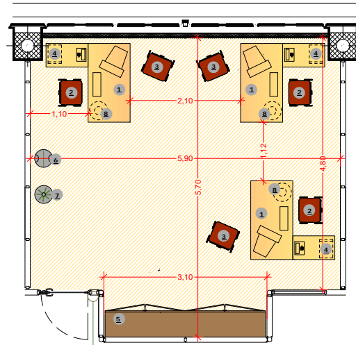
Tipologia 3 scrivanie - UFFICIO OPERATIVO - (tipo A) Mq 30,95
