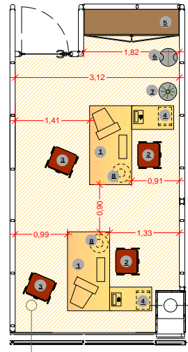
Tipologia 2 scrivanie - UFFICIO OPERATIVO - (tipo C) Mq 17,59
