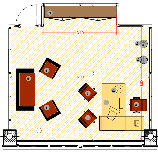
Tipologia DIREZIONALE - UFFICIO DIRIGENTE - Mq 30,95
