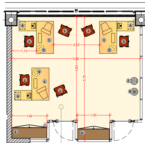
Tipologia 3 scrivanie - UFFICIO OPERATIVO - (tipo B) Mq 30,96
