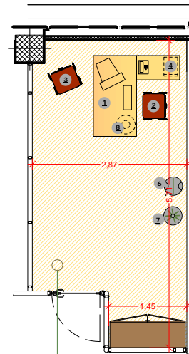
Tipologia 1 scrivania - UFFICIO OPERATIVO (tipo B)- Mq 14,76
