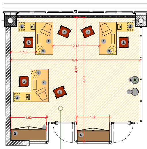
Tipologia 3 scrivanie - UFFICIO OPERATIVO - (tipo A) Mq 30,96
