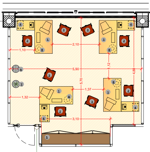
Tipologia 4 scrivanie - UFFICIO OPERATIVO- (tipo A) Mq 30,95
