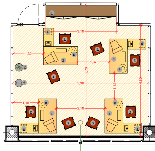
Tipologia 4 scrivanie - UFFICIO OPERATIVO - (tipo A) Mq 30,95
