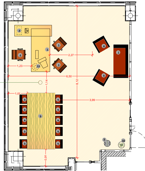
Tipologia DIRIGENZIALE - UFFICIO COORDINATORE/ ASSESSORE Mq 52,25
